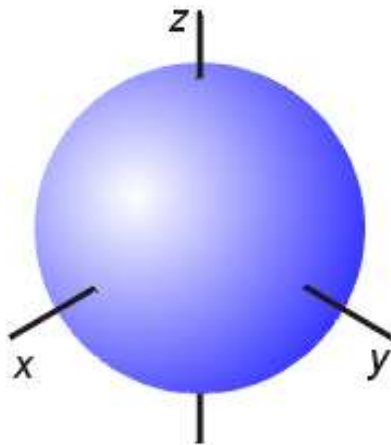
s -орбитала
