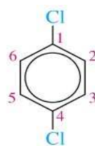
1,4-Dichlorobenzene ( p -dichlorobenzene)
