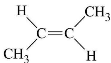
(b) trans -2-Butene
