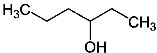
3-хексанол
