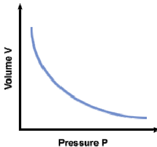
График на зависноста на волуменот од притисокот. Графикот е последица од Boyle-овиот закон
